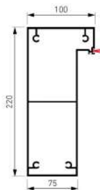
Viga P-220x100 mm • 023103
